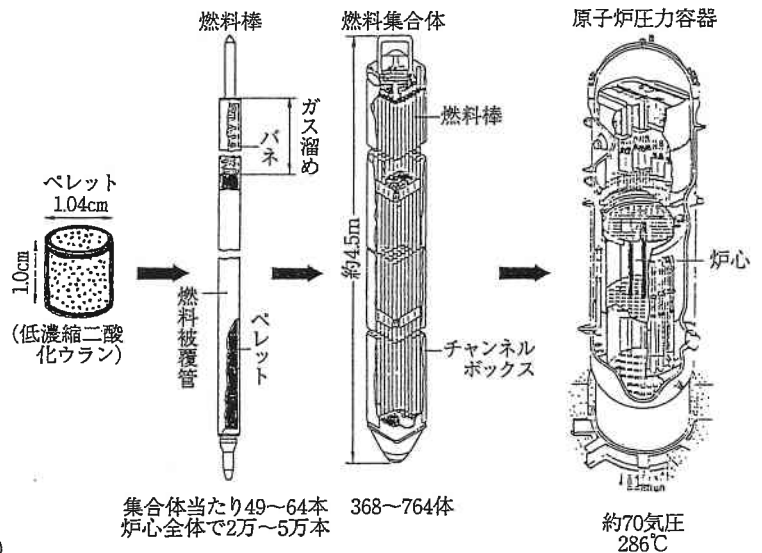
図2 沸騰水型の燃料の仕組み
