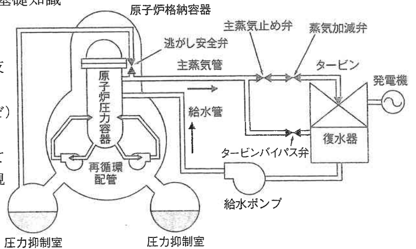
図1 事故原発（沸騰水型）の概略系統図
