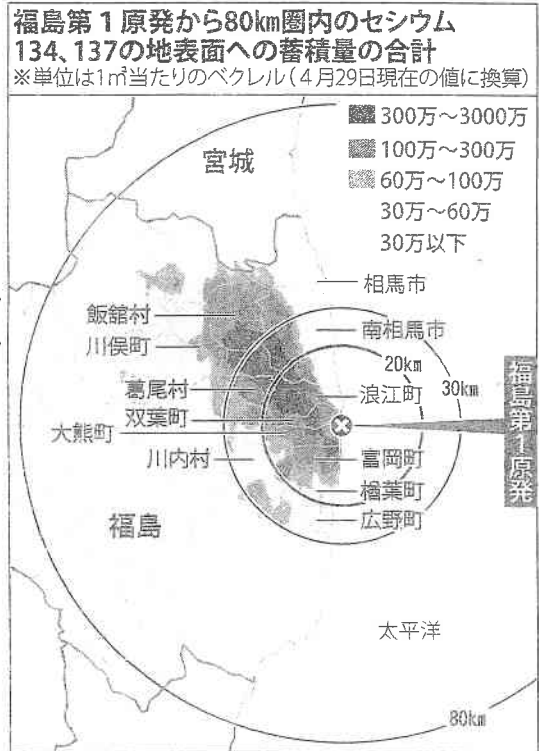
図5 放射性セシウム蓄積量の分布
